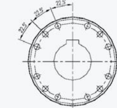
FL-14 / 12x SAE 1800
