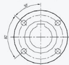
FL-11 / 4x SAE 1120, 1300, 1400 und 1500
