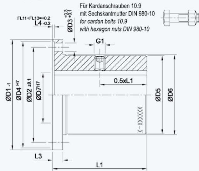
FL-11 / 4x SAE 1120, 1300, 1400 und 1500
