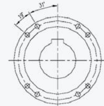
FL-13 / 8x SAE 1880
