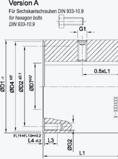
FL-11 / 4x SAE 1120, 1300, 1400 und 1500
