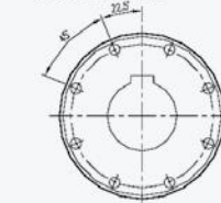
FL-12 / 8x SAE 1600, 1700 und 1900
