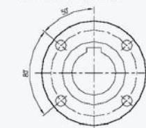
FL-11 / 4x SAE 1120, 1300, 1400 und 1500
