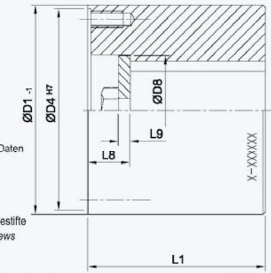
FL-13 / 8x SAE 1880
