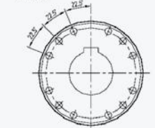
FL-14 / 12x SAE 1800
