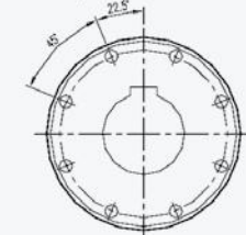
FL-12 / 8x SAE 1600, 1700 und 1900
